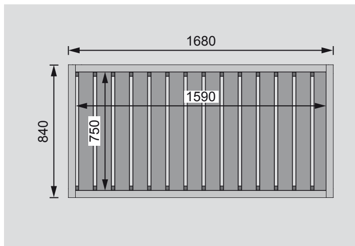
Draufsicht (in mm)
